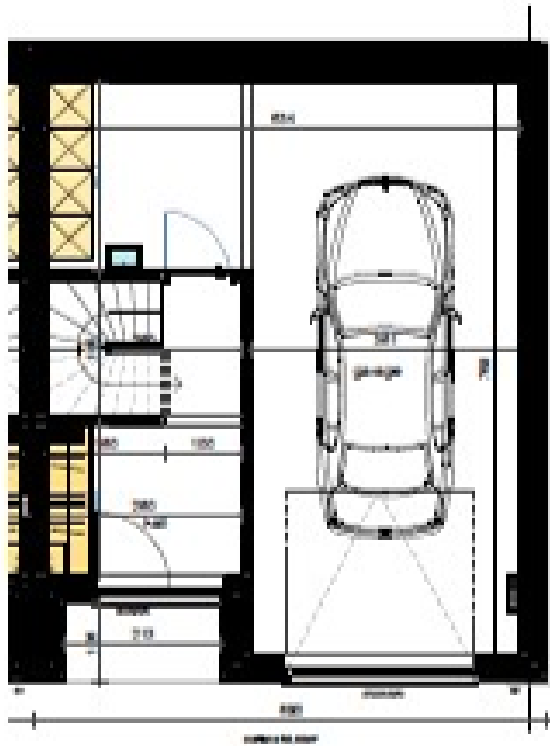
sous-sol 1:100
